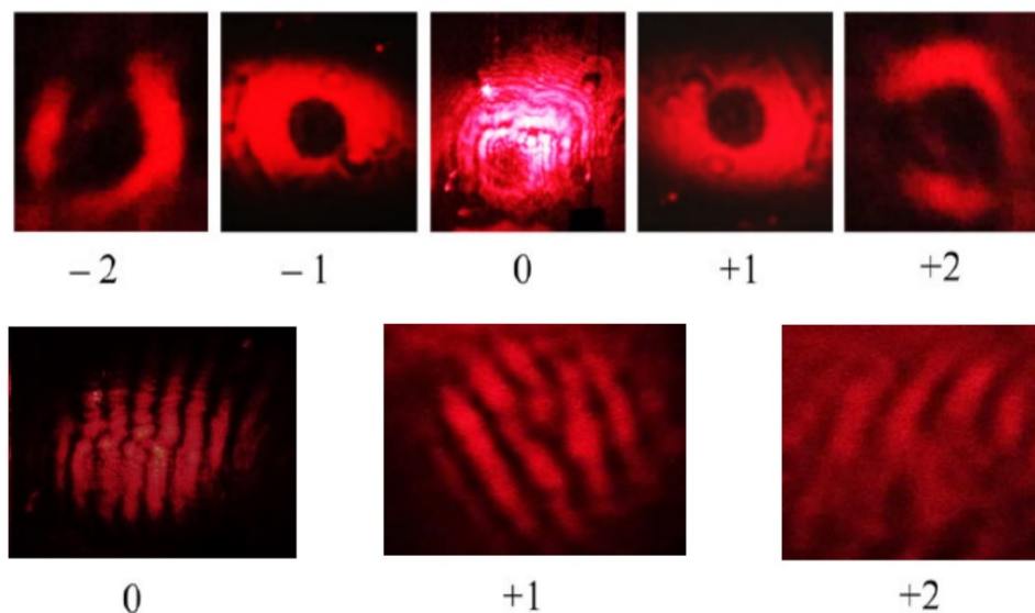
Fig. 18: Imaginile secțiunilor transversale ale fasciculelor de lumină în ordinele de difracție de la -2, până la +2 (rândul de sus) și rezultatele sumării interferometrice a ordinelor 0, +1 și +2 cu o undă plantă [42].
