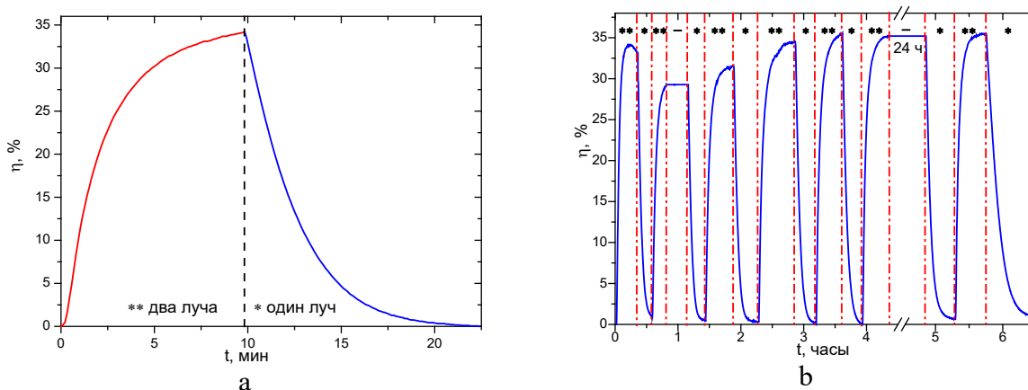
Fig. 17: Cinetica modificării ED în timpul expunerii holografice a structurii \text{As}_2\text{S}_3 -Se cu două fascicule cu polarizare LCP:RCP: (a) - până la atingerea valorii maxime (** - înscrierea RD, * - ștergerea RD după stoparea unui fascicul, (b) - înscrierea și ștergerea ciclică a RD (7 cicluri). Segmentele "-" corespund stocării RD, atunci când ambele fascicule sunt stopate [40].
