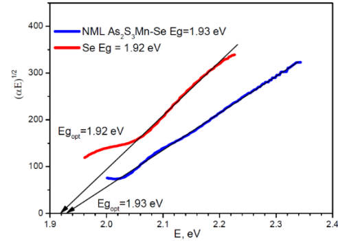
Fig. 6. Graficul dependenței (h\nu\alpha)^{1/2} versus h\nu pentru structura multistrat \text{As}_2\text{S}_3\text{:Mn-Se} și stratul de Se [11].
