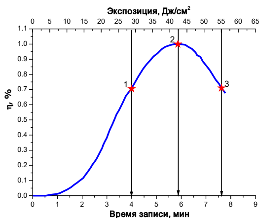
Fig. 8. Cinetica modificării ED în rețelele înregistrate în filmul \text{As}_2\text{S}_3 la diferite doze: 1 - subexpusă; 2 – normal expusă; 3 – supraexpusă [23].
