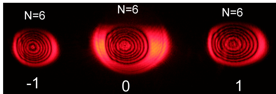
Fig. 12. Tabloul de difracție pentru maximele de ordinul zero și întâi cu inele observate în fiecare ordin (câte 6 inele) [29]
