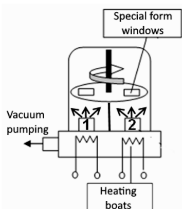
Fig. 1. Atașament pentru depunerea structurii multistrat pe bază de SC cu două evaporatoare: 1 – pentru \text{As}_2\text{S}_3 ; 2 – Se [6].
