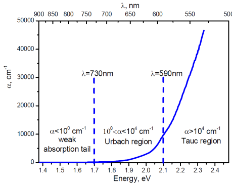
Fig. 5. Spectrul de absorbție optică al structurii multistrat \text{As}_2\text{S}_3\text{:Mn-Se} cu trei regiuni majore [11].
