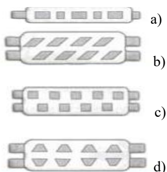
Figura A 4.6. Variante de trasare a fâșiilor din piele cu rol decorativ. (a) dintr-o fâșie (ornament pătrat), (b), (c), (d) din două fâșii
