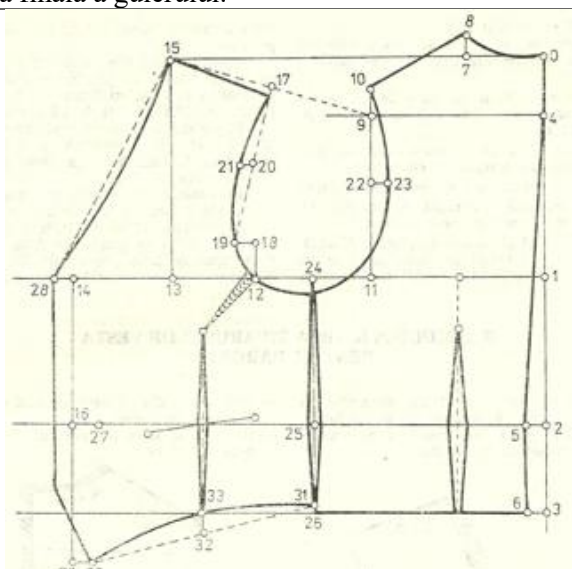
Figura A 6.3. Reprezentarea tiparului de bază și tiparului de model pentru modelul bundiță din piele naturală
