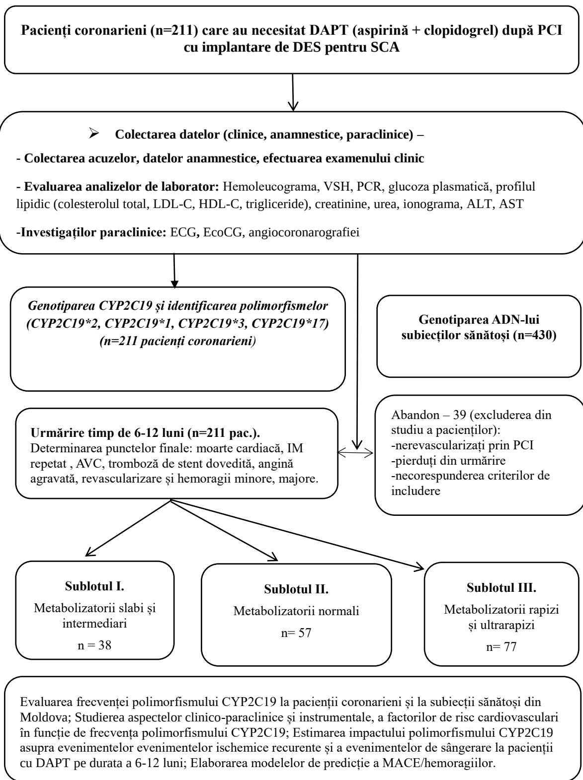
Figura 2.2. Design-ul cercetării
