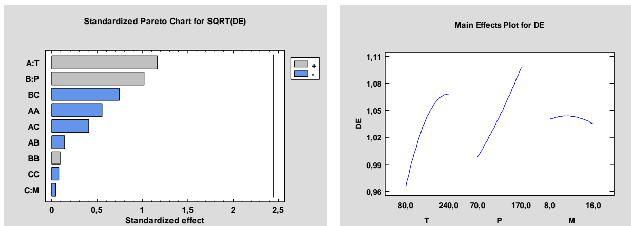
Fig. 4.11. Diagrama Pareto și graficul efectelor temperaturii și presiunii densificării și a conținutului de umiditate
